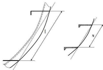
그림 1.2 곡부재에 대한 늑골 스패(왼쪽) 및 늑골 간격(오른쪽)의 정의
