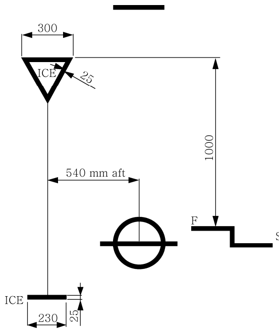
그림 1.1 빙흘수 표시
