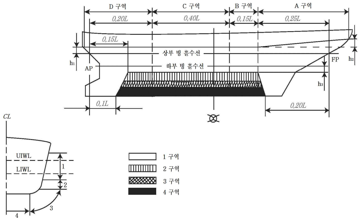
그림 3.8 쇄빙선의 대빙구역
